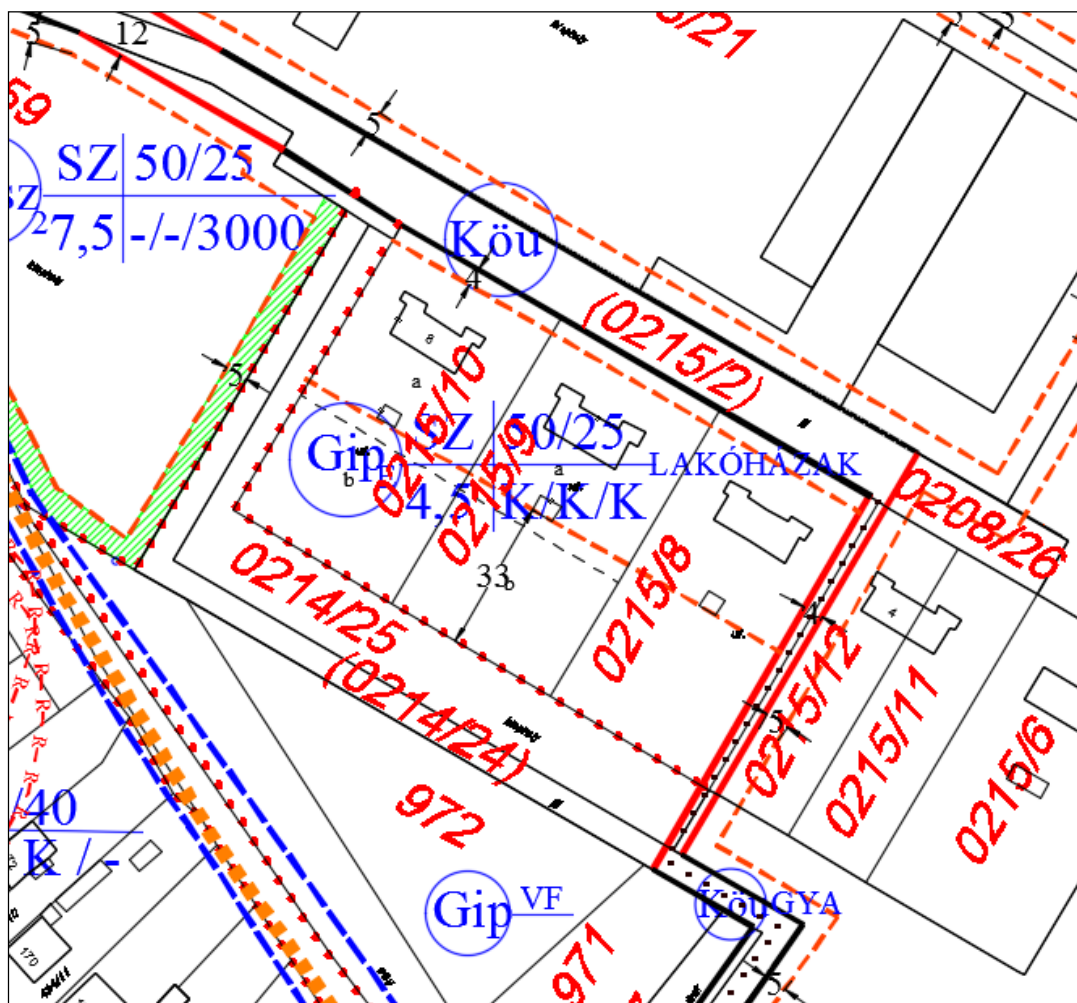
Kivágat a hatályos szabályozási tervből
