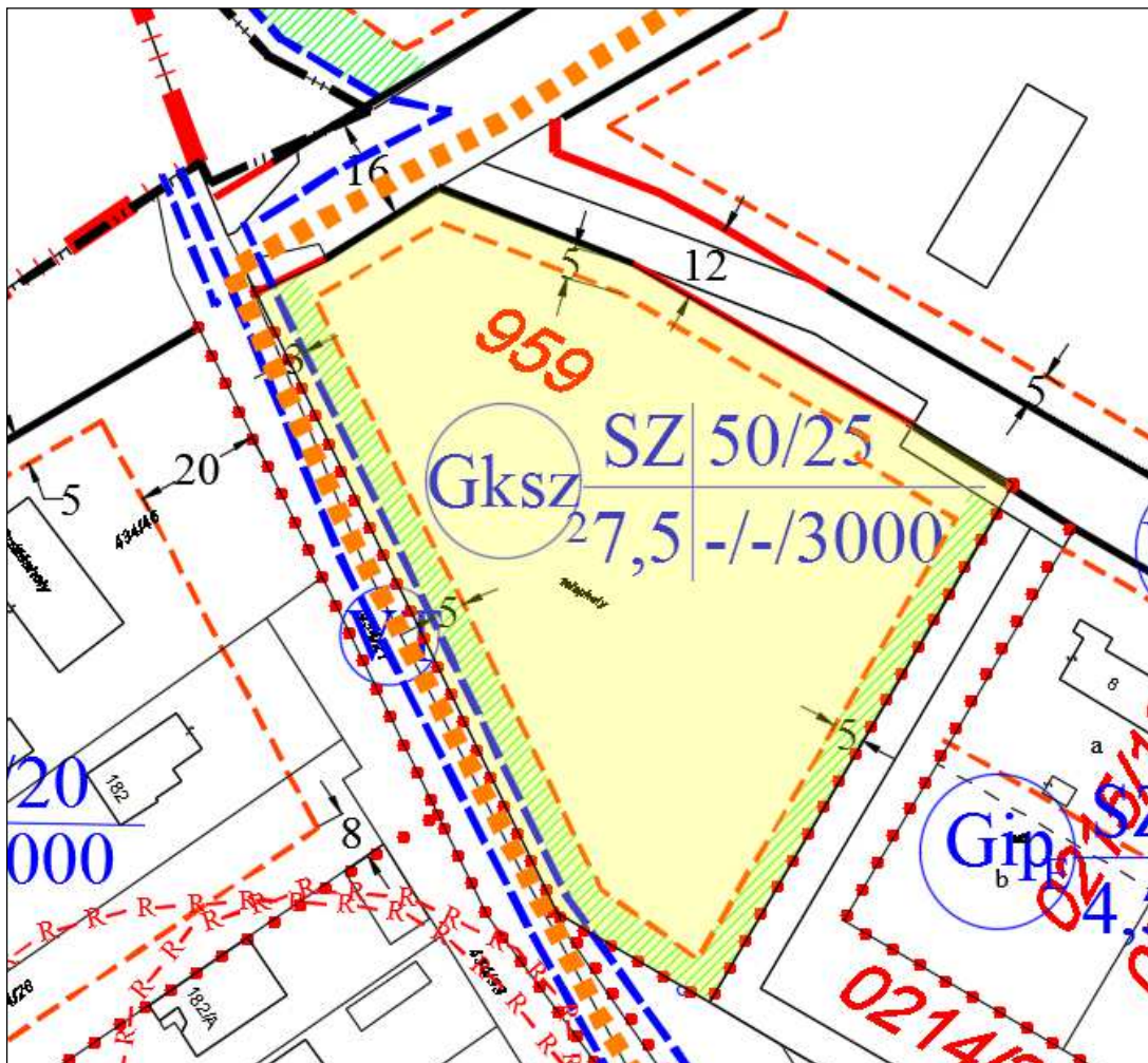
Kivonat a hatályos szabályozási tervből – 959 hrsz Gksz2 övezet
