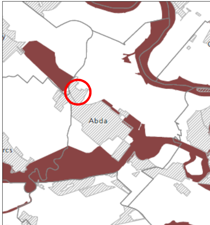
Kivonat a Győr-Ménfőcsanak Vármegyei TRT-ből Külfejtéses bányatelek kijelölésének korlátozásával érintett területek övezete
