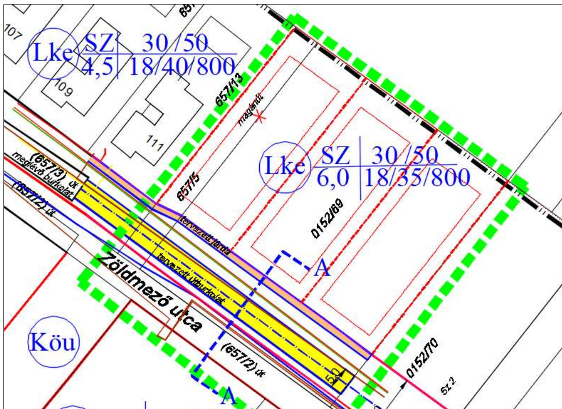
A Zöldmező utca a javasolt helyszínrajzi elrendezése
